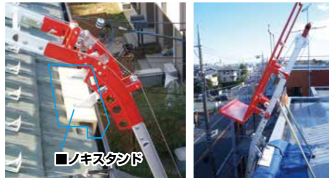
■極小曲りレール特殊使用例
