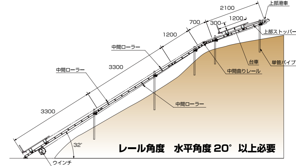
■標準台車 : 台車寸法 (H750×W650×D300) ■ロング台車 : 台車寸法 (H1200×W650×D300)
