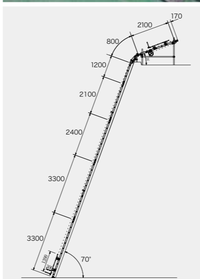
【斜め設置】竹田城跡の石垣改修工事での設置例 単管パイプで槽を組んでレールの固定をした仕様
