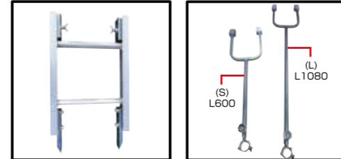
■中間レール (レール幅400mm) 0.6m、1.2m、1.8m 2.4m、3.0m
