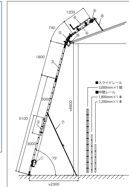
UP100S (ショートレール)
